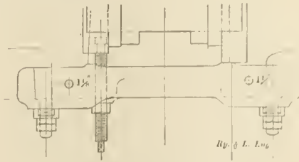
M. C. R. R. PEDESTAL BINDER.
